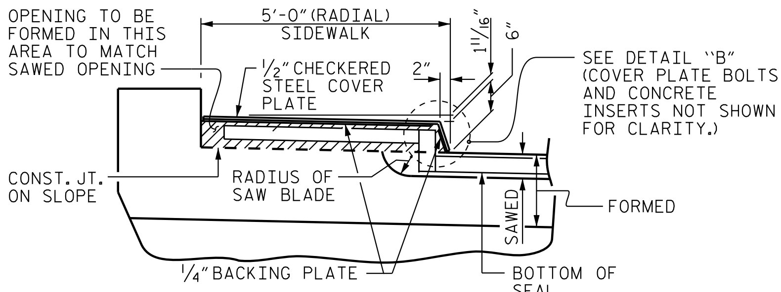
SECTION D-D
